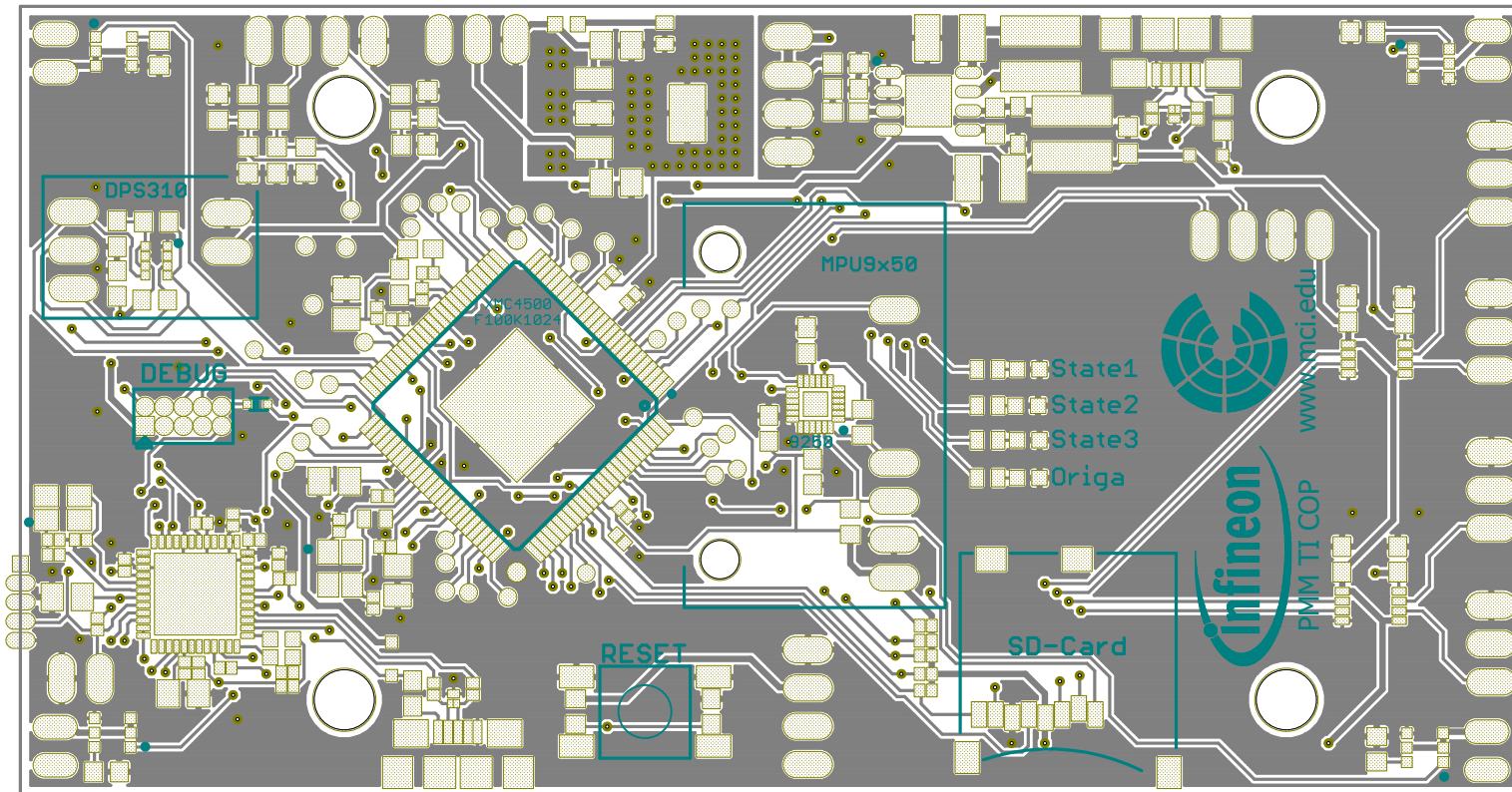
Layer 1 TOP
